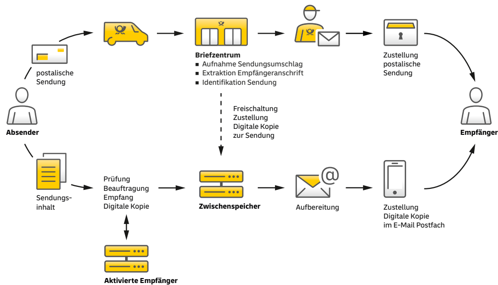
Abb. 9: Schematische Darstellung des Ablaufs zur Zustellung der Digitalen Kopie
